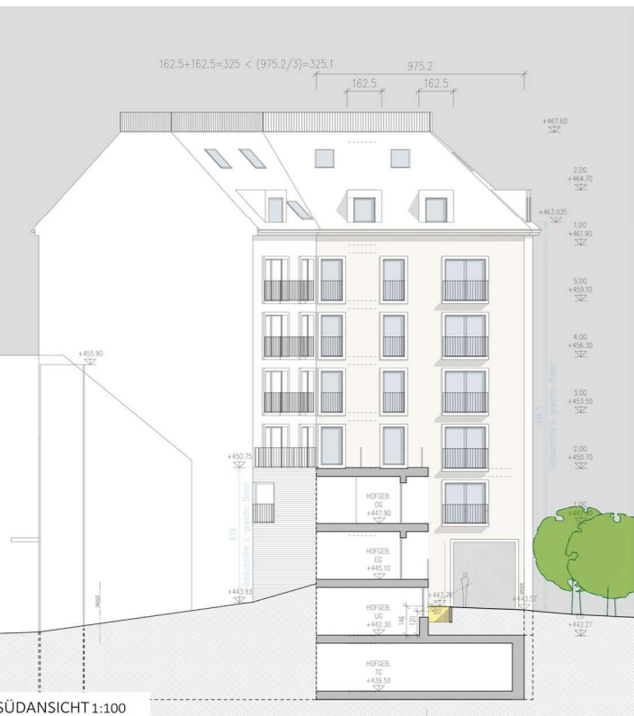
SÜDANSICHT 1:100
